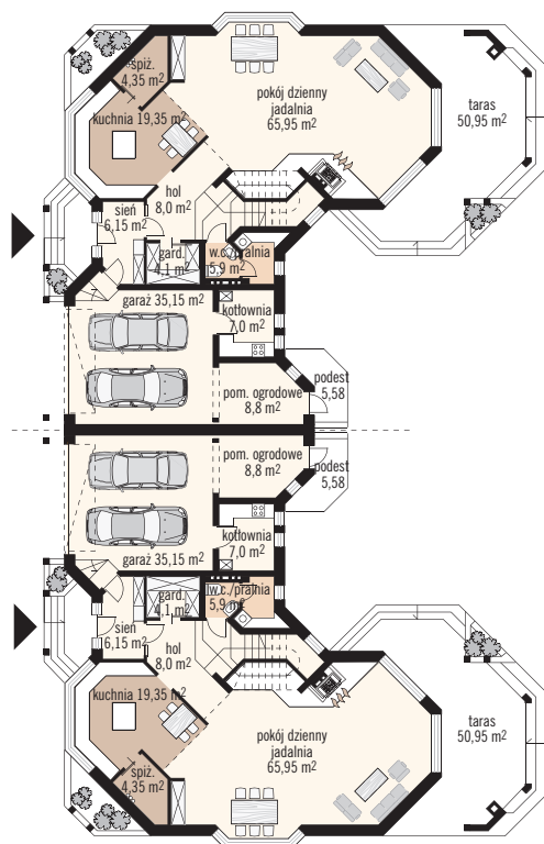
parter: 164,75 m 2 – jeden segment
