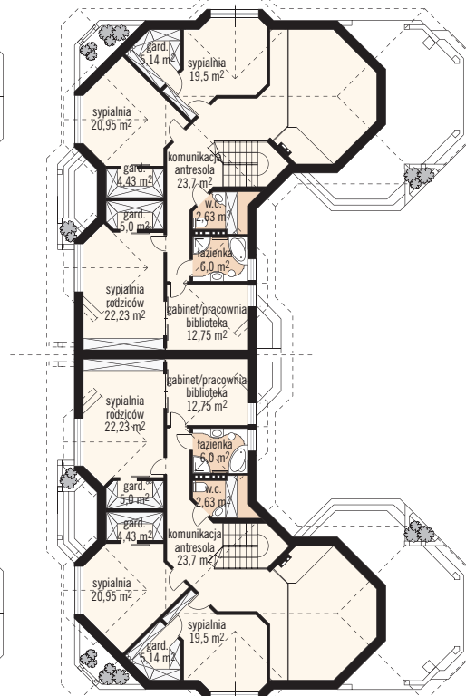
poddasze: 122,33 m 2 – jeden segment
